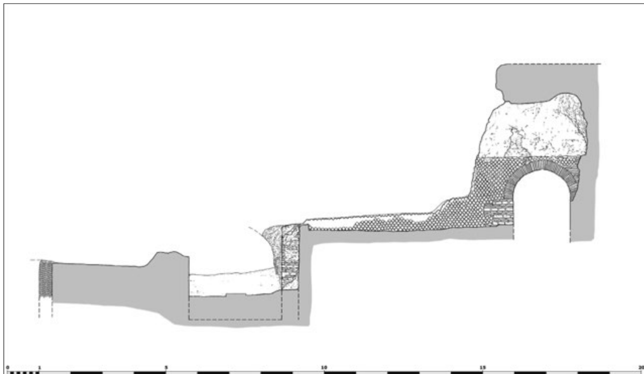
Fig. 10. Formia, anfiteatro. Sezione nord-sud dei resti murari portati in luce fino al 2012 (rilievo AION s.n.c.).
